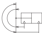
Symbol graficzny Chwytek dwustronnego działania
