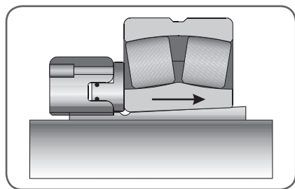
图11. 一个滑动面
