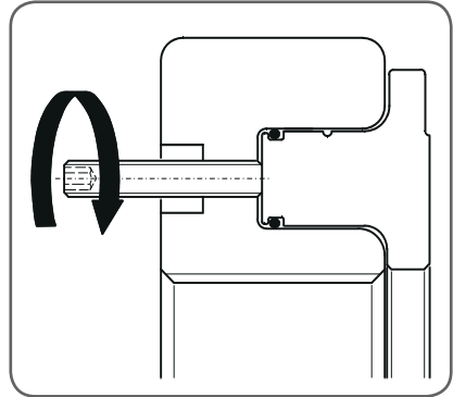
Figuur 15. De zuiger wordt uit de ring geduwd
