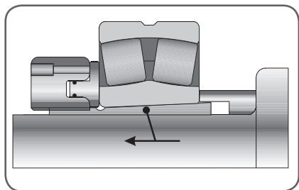
Figur 12. Två glidytor
