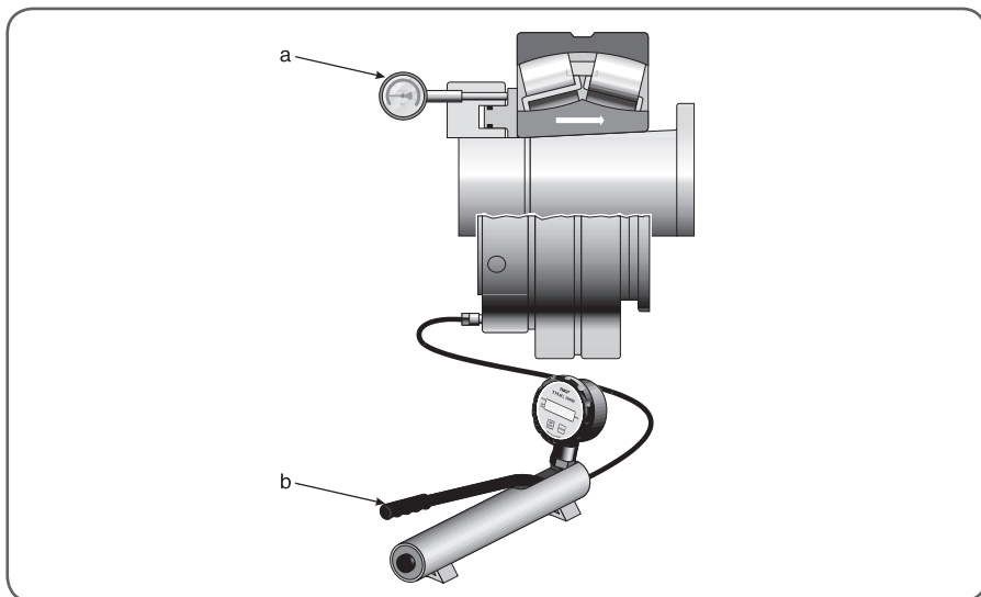
Figuur 9. Meetklok en hydraulische pomp
