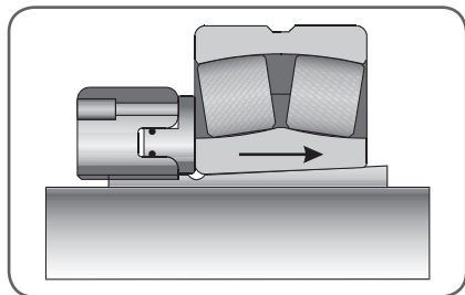
Figur 11. En glidyta
