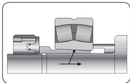
Figur 13. Två glidytor
