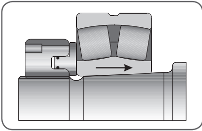
Figuur 10. Eén schuifoppervlak
