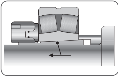
Figuur 12. Twee schuifoppervlakken
