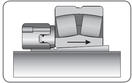
Figuur 11. Eén schuifoppervlak
