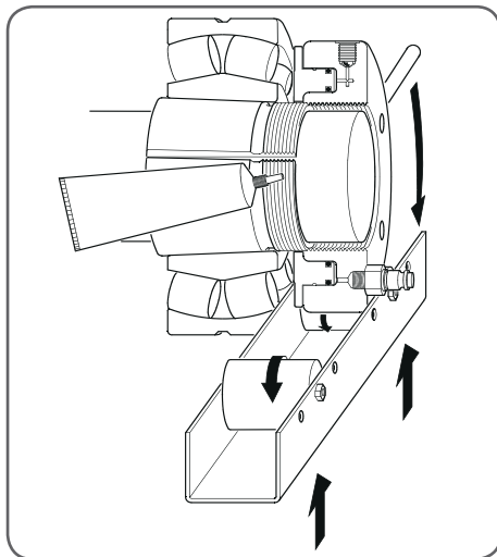
Figur 2. Stöd för en stor hydraulisk mutter
