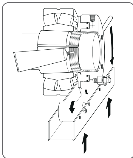
Figure 2. Ondersteuning voor een grote hydraulische moer
