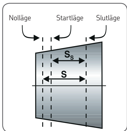
Figur 14. Lagerlägen
