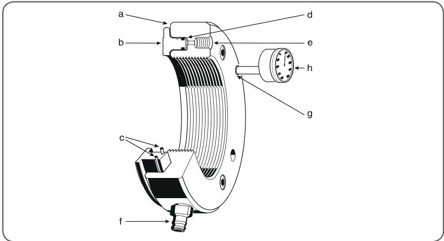
Figuur 1. Onderdelen van de hydraulische moer
