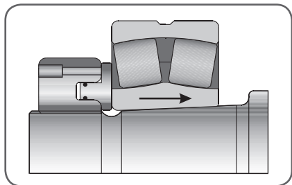
Figur 10. En glidyta
