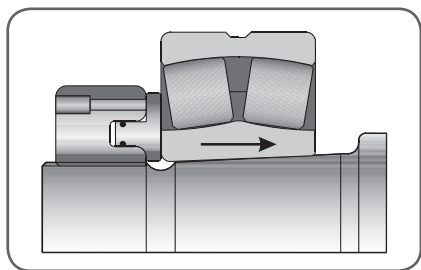
图10. 一个滑动面
