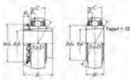
UK3...D1;H, HA, HE, HS
